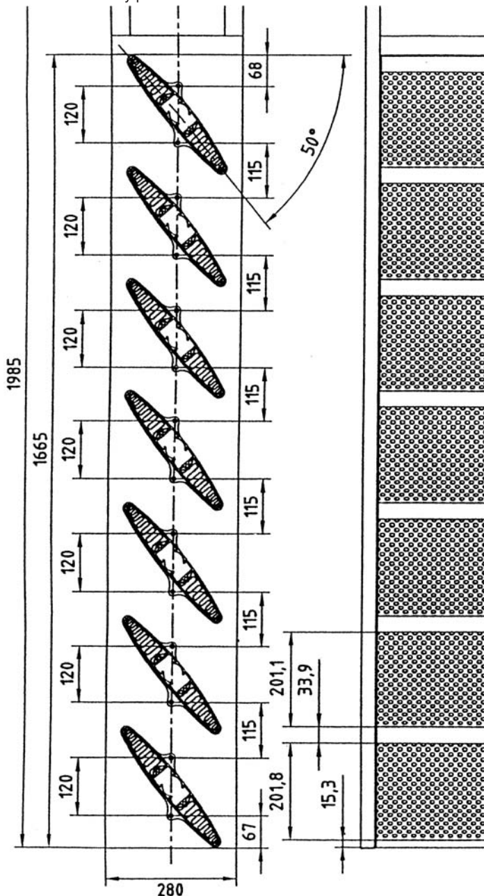
Posazení lamely při sklonu 50°
