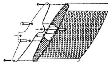
Ocelová koncovka při sklonu 50°
